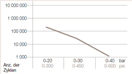
Druckbelastung
