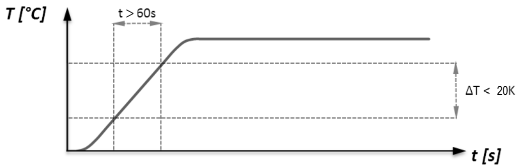
Abbildung 6: Maximale Temperaturänderung beim Hochfahren zum Erreichen des Beharrungszustandes zur Vermeidung von Thermospannungen ( < 0,33K/s )
