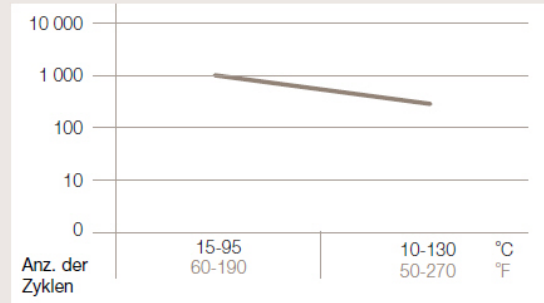
Thermische Belastung
